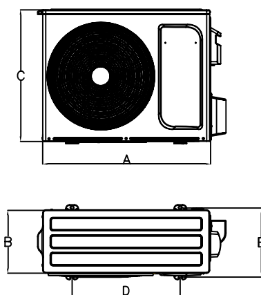
Наружный блок
