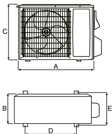
Наружный блок
